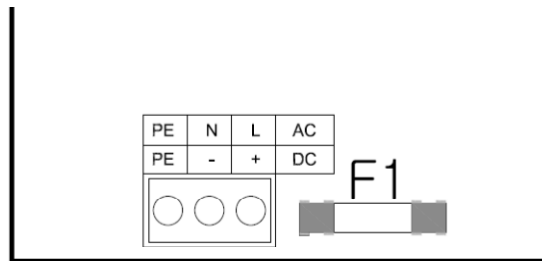
Abbildung 6. Anschluss der Stromnetzkabel
