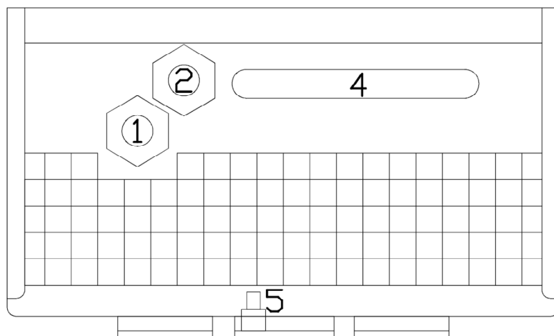
Figura 2 Vista de la parte inferior de la carcasa que muestra las entradas de cable: modelos de tres salidas
