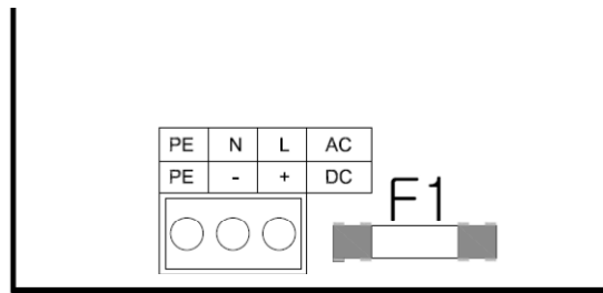
Figura 6 Conexión de la red eléctrica
