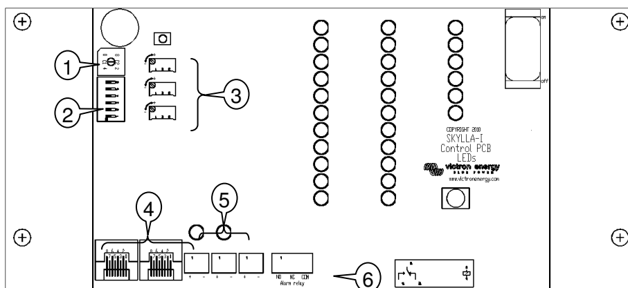
Figure 7 Connexions et contrôles internes
